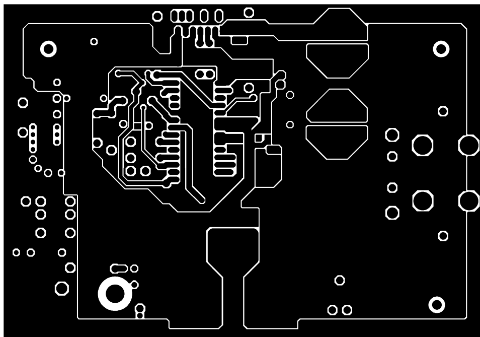
Figure 25. Top Layer
