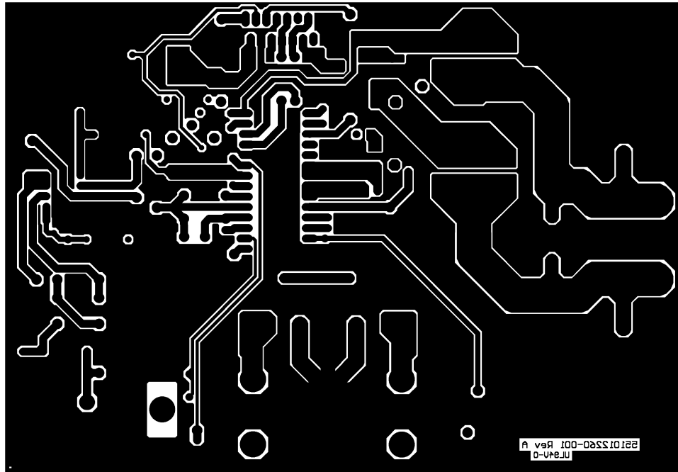
Figure 26. Bottom Layer
