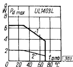
Dopuszczalna moc strat w funkcji temperatury otoczenia
