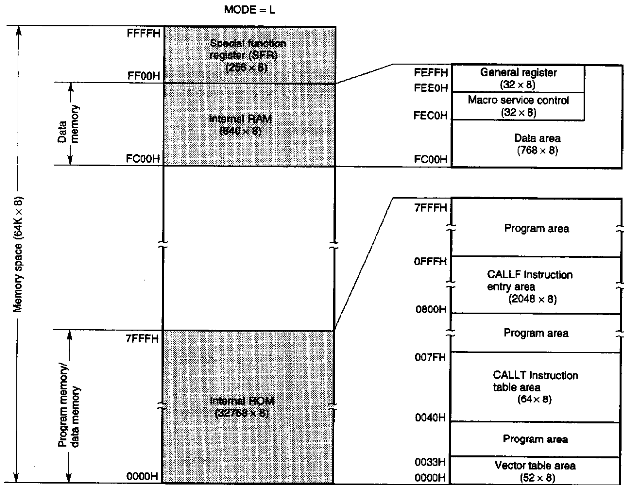
Fig. 2-2 Memory Map (μPD78148)
