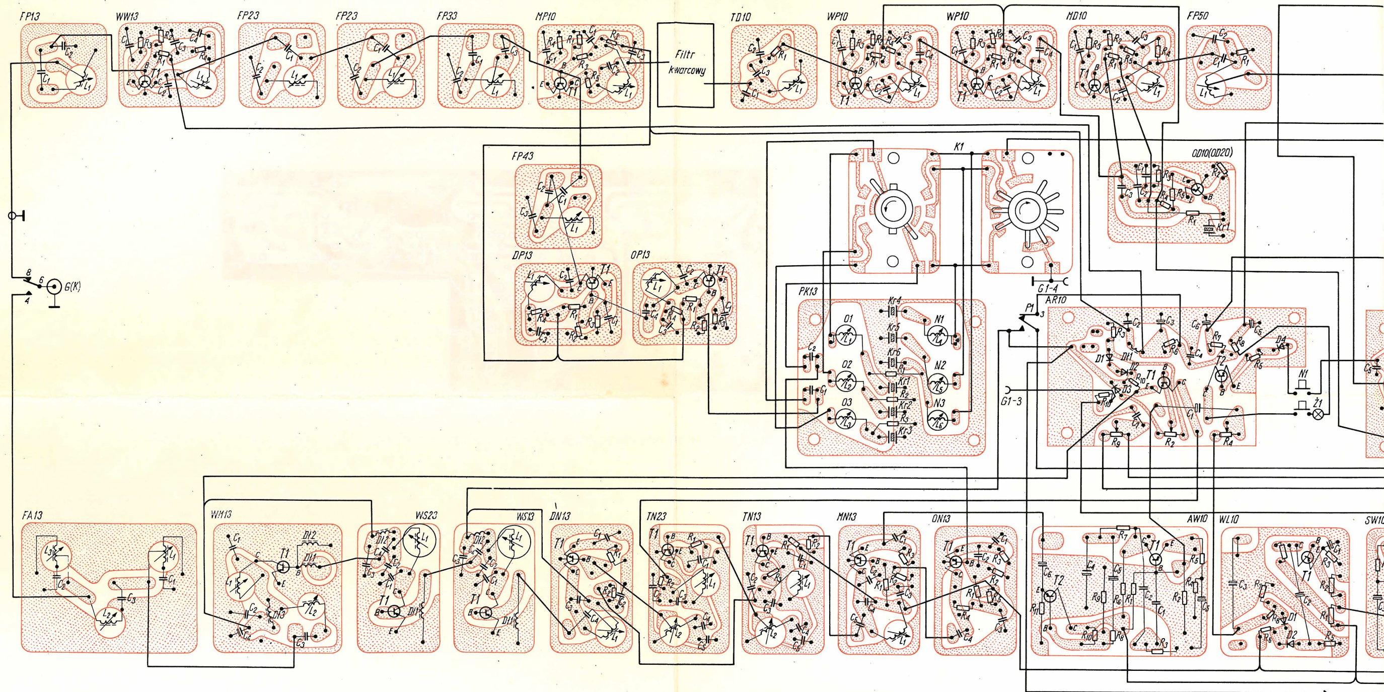
Rys. 8-3. Schemat połączeń elementów i obwodów drukowanych poszczególnych modułów radiotelefonu FM-315
