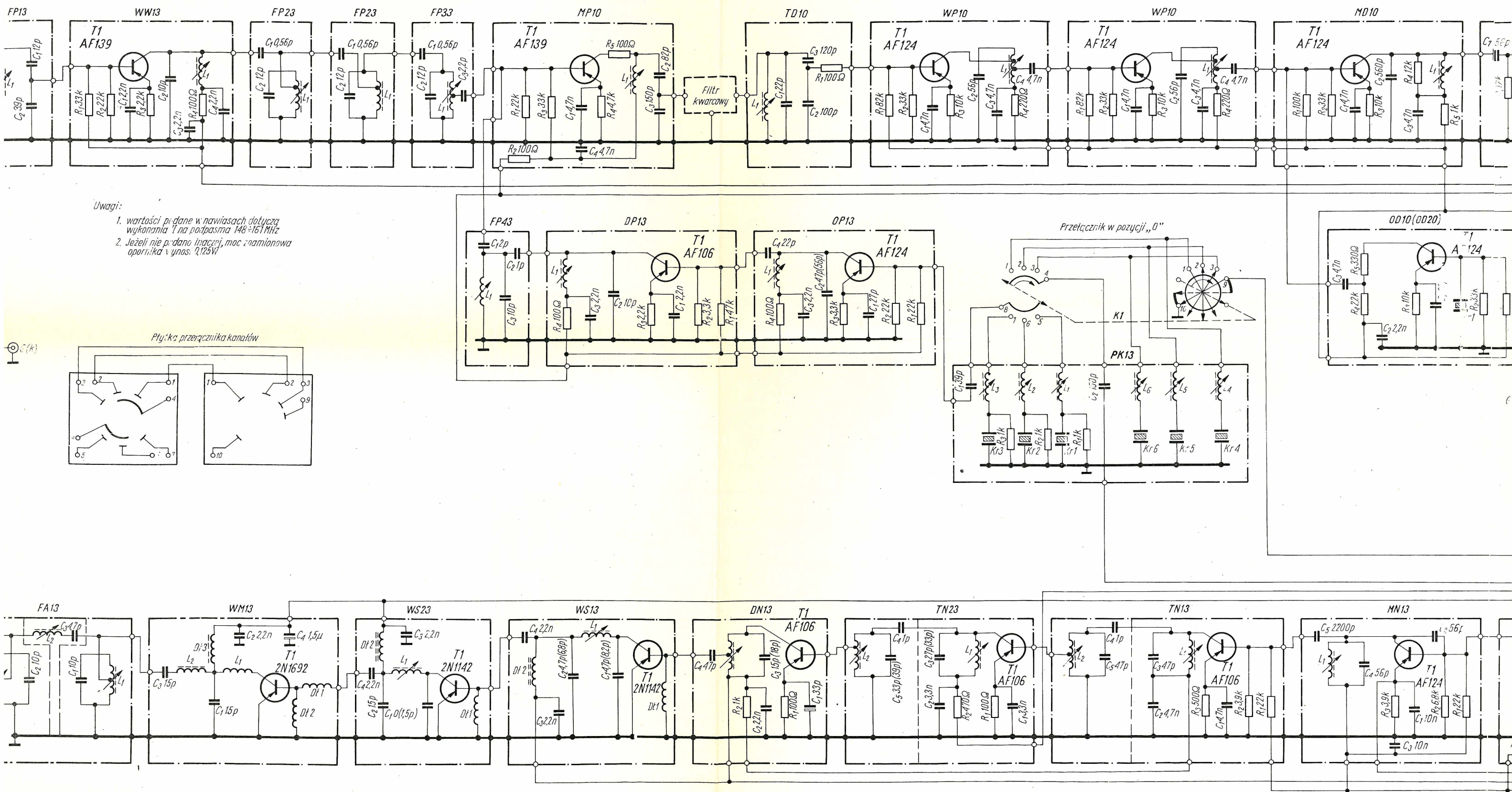
Schemat zespołu nadawczo-odbiorczego radiotelefonu FM-315
