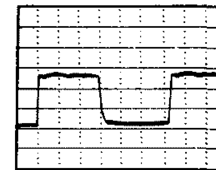
⑬ 6,4 Vp-p Horiz.
